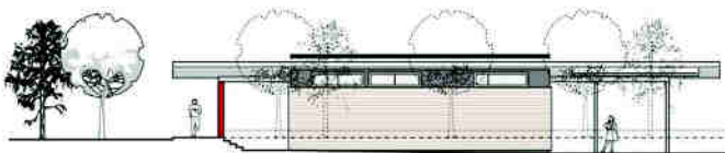
ANSICHT NORD
